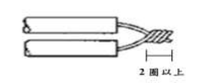
圖一五~九 實心線終端連接法
