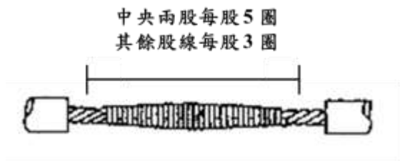
圖一五~三 絞線直接連接法
