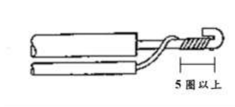
圖一五~十 不同線徑之實心線終端連接法
