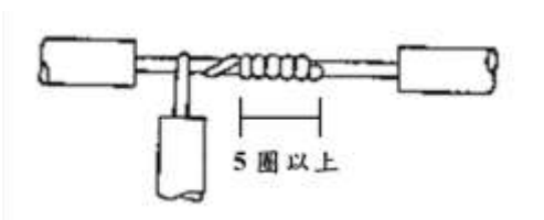
圖一五~五 實心線分歧連接法
